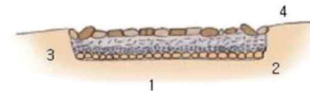
| 로마도로의 기초공사 |
